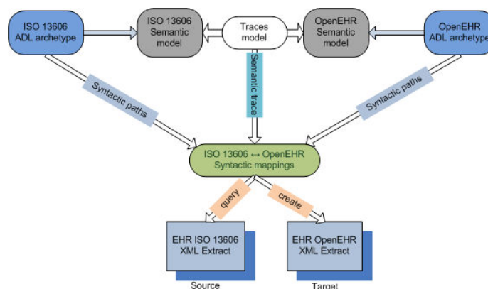
Fig. 1. Esquema de transformación de datos
