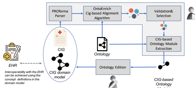
Fig. 4. Diagrama de procesamiento del contenido de la guía clínica comput-erizada
