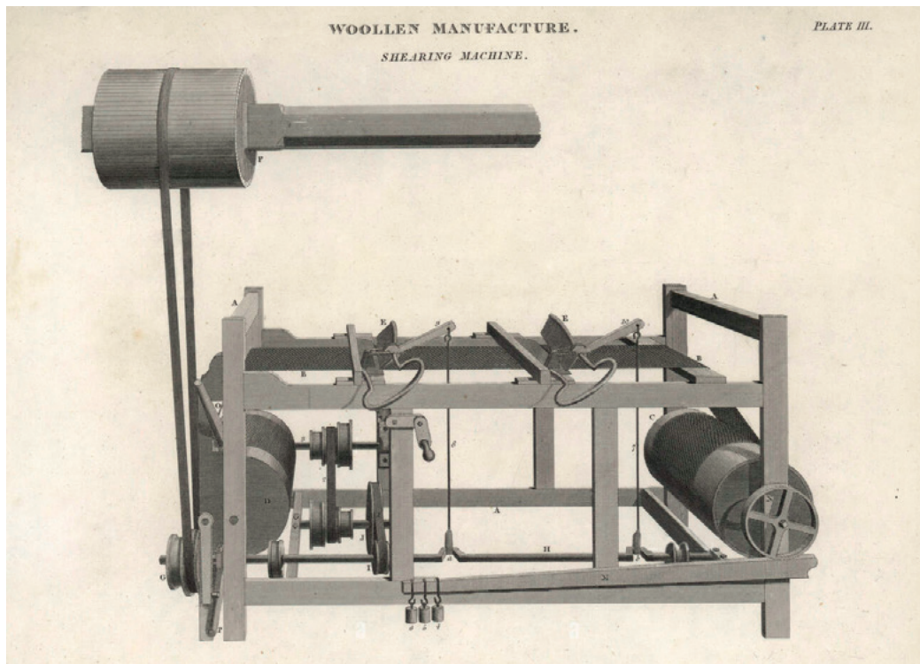
Fig. 3: Màquina de tondre "shearing frame" amb dues tisores. Gravats de Wilson Lowry segons una il·lustració de J. Farey de la Cyclopaedia or Universal Dictionary d'Abraham Rees , Londres, 1811.
