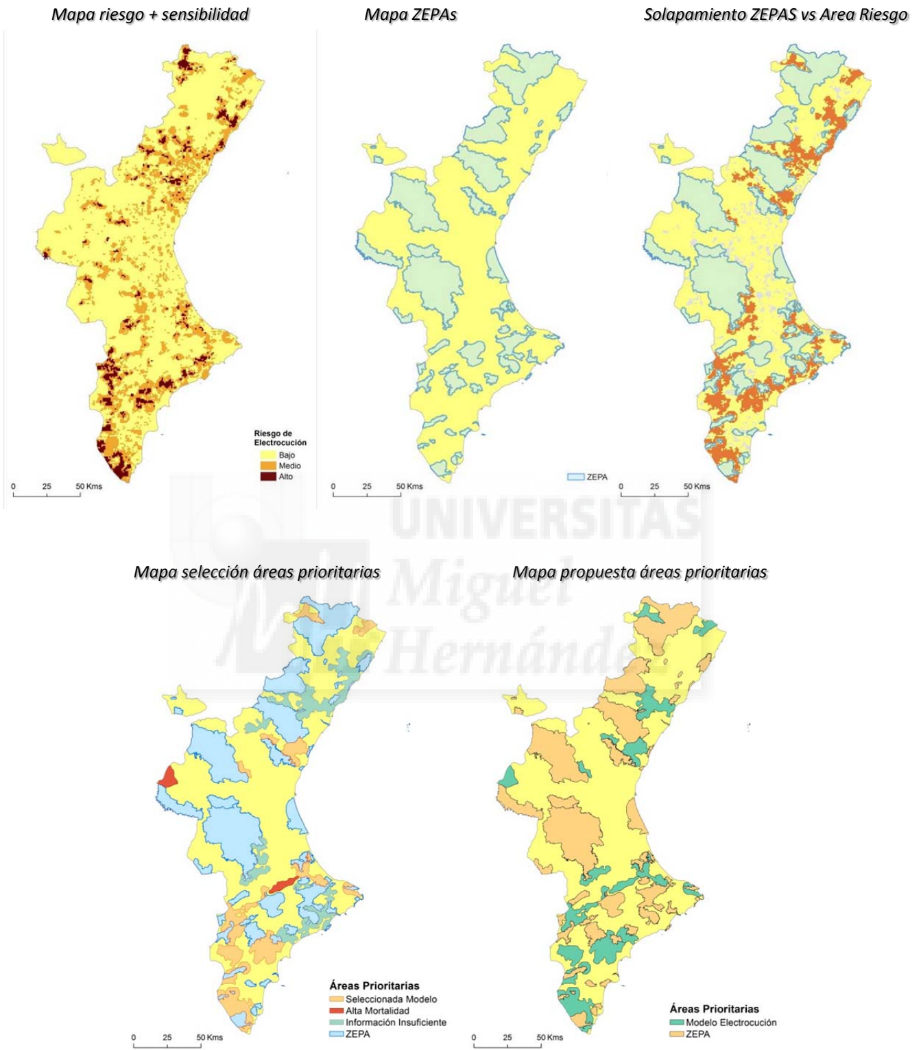
Figura 3.6. Solapamiento de las zonas con alto valor de riesgo de mortalidad y de sensibilidad (a) y las zonas de especial protección para las aves ZEPAS (b). Localización de las áreas prioritarias propuestas por el modelo, las áreas con información insuficiente y las áreas seleccionadas por mortalidad. Propuesta final de áreas prioritarias contra la electrocución
