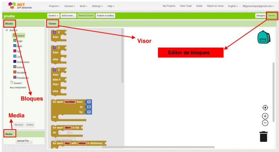
Ilustración 20: Interfaz "Editor de bloques". MIT App Inventor 2.
