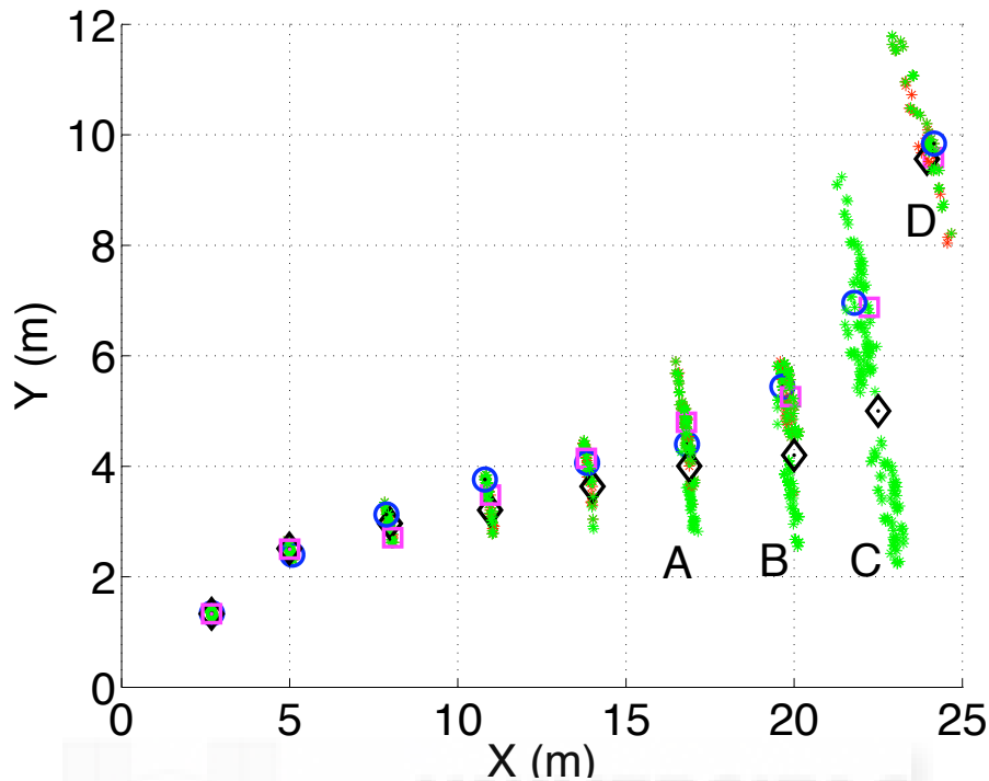
Figura 2.11: Ejemplo de diferentes estimaciones del camino del robot. Con círculos (○) se indica el camino real del robot. La estimación según 2.61 se indica con cuadrados (□) y la ecuación (2.60) se indica con diamantes (◇).
