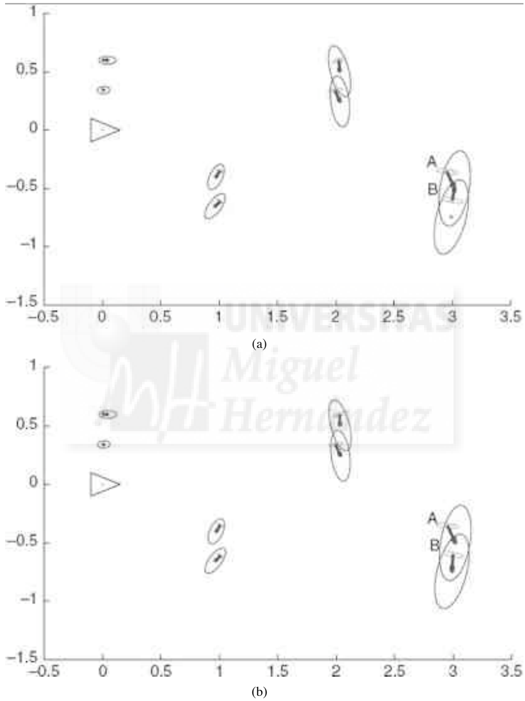
Figura 2.4: Diferentes alternativas para la asociación de datos en un caso concreto.
