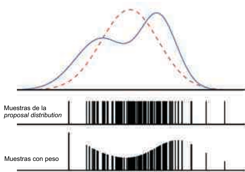
Figura 2.10: Ejemplo de la utilización de SIR. En rojo la proposal distribution . En azul la target distribution .
