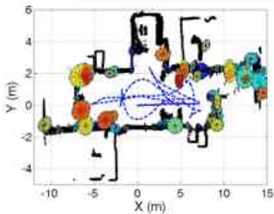
Figura 4.15: En la figura (a) se presenta una vista 2D de un mapa visual. En la figura (b) se presenta el mismo mapa visual superpuesto con un mapa creado a partir de los datos de láser. En la figura (c) se presenta una vista 3D del mapa.
